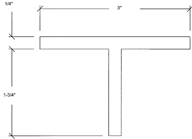
FRP T ASTRAGAL
